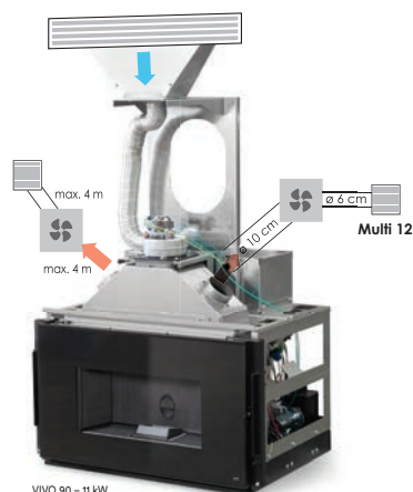
VIVO 90 - 11 kW
