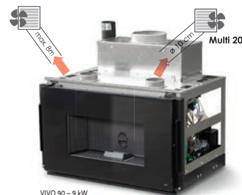
VIVO 90 - 9 kW
