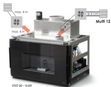
VIVO 90 - 9 kW
