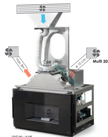
VIVO 90 - 11 kW
